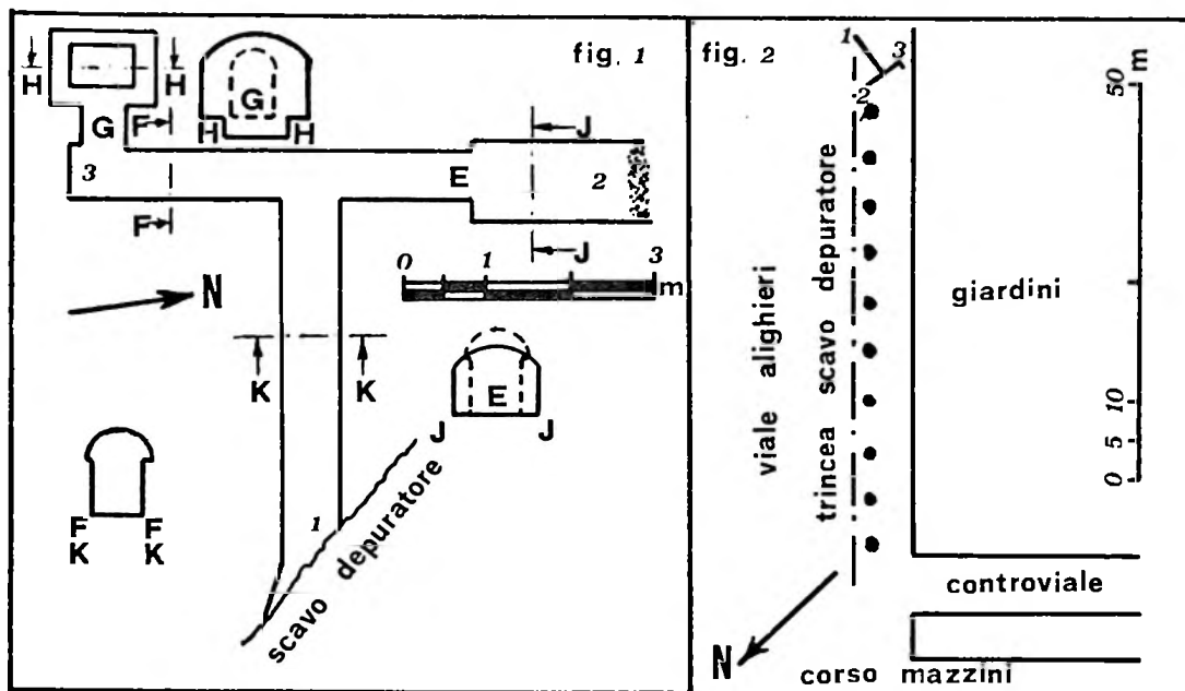
Ubicazione, rilievo planimetrico e sezioni trasversali dei ritrovati cunicoli con Fornelli di mina della «Piazza d'Armi S.Croce» (ril. di R. Massucco e Sergio Sdobba, S.S.S.P.-G.S.S.).
